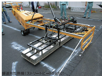
舗道用加熱機(ストリートヒートSR60)
